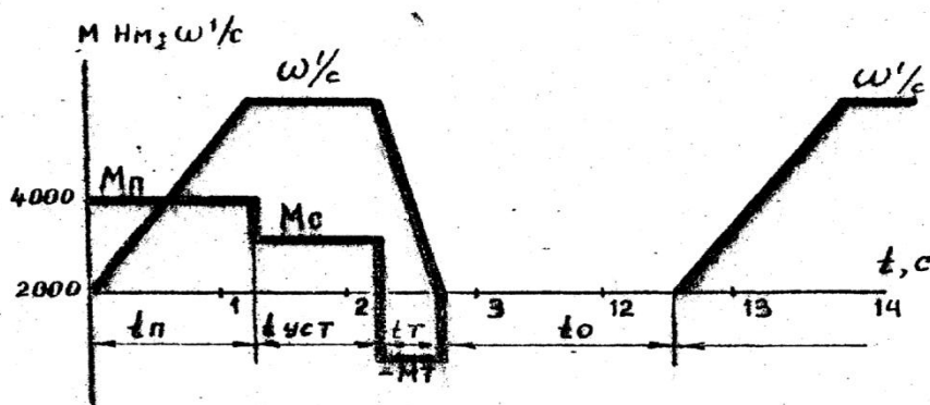
Рисунок 2.4 Діаграма навантаження
