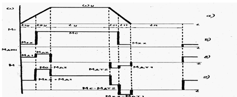
Рисунок 2.3 - Швидкісна діаграма (а), навантажувальна діаграма (б), діаграма динамічних моментів (в) і навантажувальна діаграма двигуна (г)
